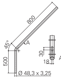
LMW 48 - 500/800 - FT
