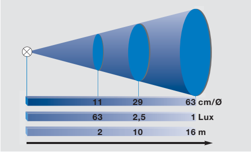
Range-diagram HE 5 EN
