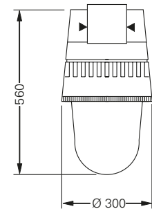
EV ... 150 - 250 ZM
