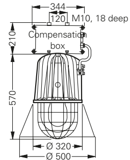
dHLS 85 ... comp.
