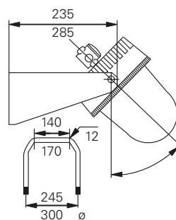
SPEV 200/500
