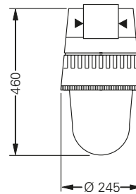
EV ... 70 - 125 ZM
